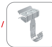
Зажим балочный 3-8/8-14мм под трубу ZB3-8-Tr20-25/ ZB8-14-Tr25/ ZB8-14-Tr25
