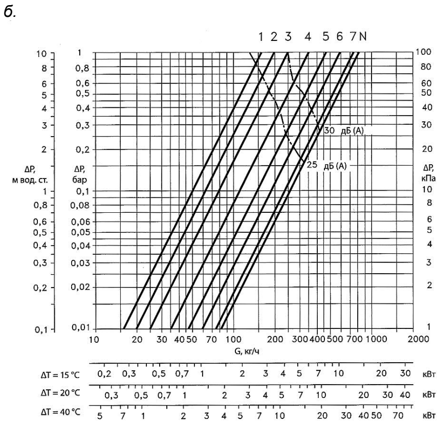
Рис. 2.3. Гидравлические характеристики терморегуляторов «Данфосс» RTR-N 15 (а) и RTR-N 20 (б), предназначенных для двухтрубных систем отопления (при различных уровнях монтажной настройки клапана)
