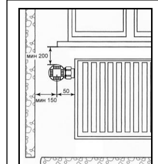
Рис. 5.5. Размещение терморегулятора
