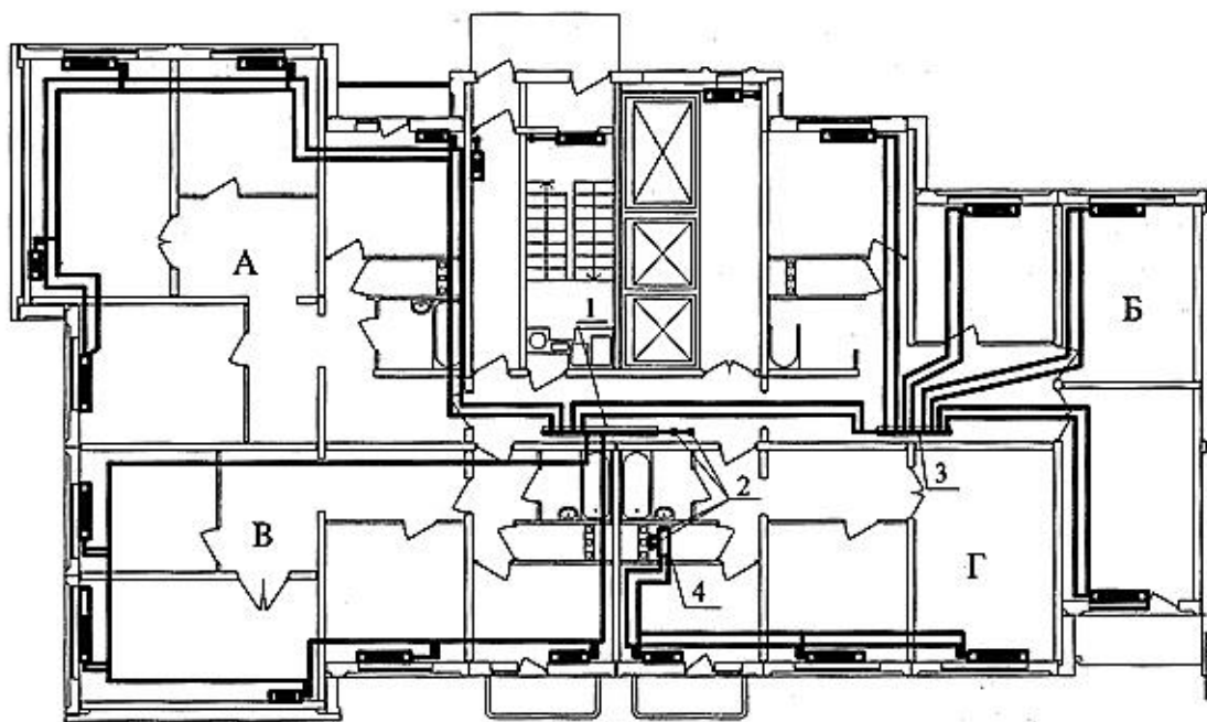
Рис. 1.11. Поквартирные системы отопления с горизонтальной разводкой теплопроводов: А – периметральная двухтрубная с этажным узлом регулирования и учёта теплоты; Б- радиальная двухтрубная с этажным узлом регулирования и учёта теплоты; В – периметральная однетрубная с этажным узлом регулирования и учёта теплоты; Г – периметральная двухтрубная с квартирным узлом регулирования и учёта теплоты; 1 – этажный узел регулирования и учёта теплоты, 2 – стояки, 3 – коллектор, 4 – квартирный узел регулирования и учёта теплоты
