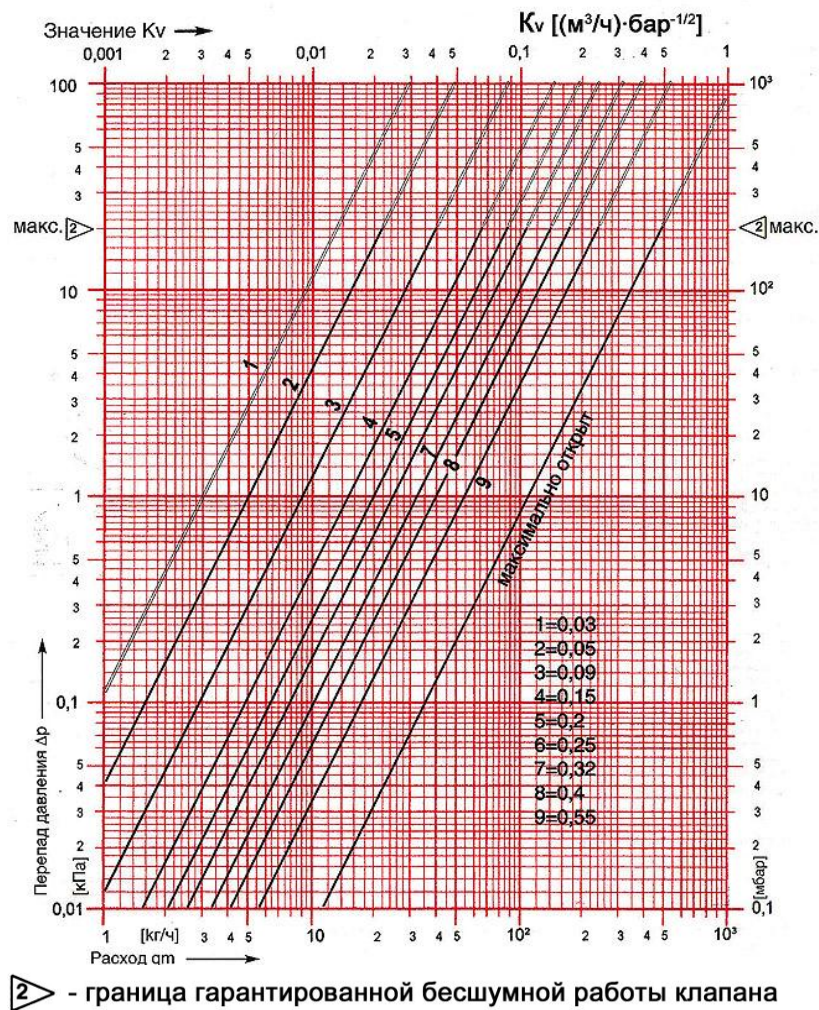
Рис. 2.2. Гидравлические характеристики термостатов « HERZ-TS-90-V » с присоединительными размерами 3/8" и 1/2" с настройкой на режим 2К (2°C) и при снятом термостатическом элементе (при полном открытии клапана)
