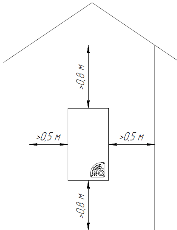
Рисунок 3. Схема установки
