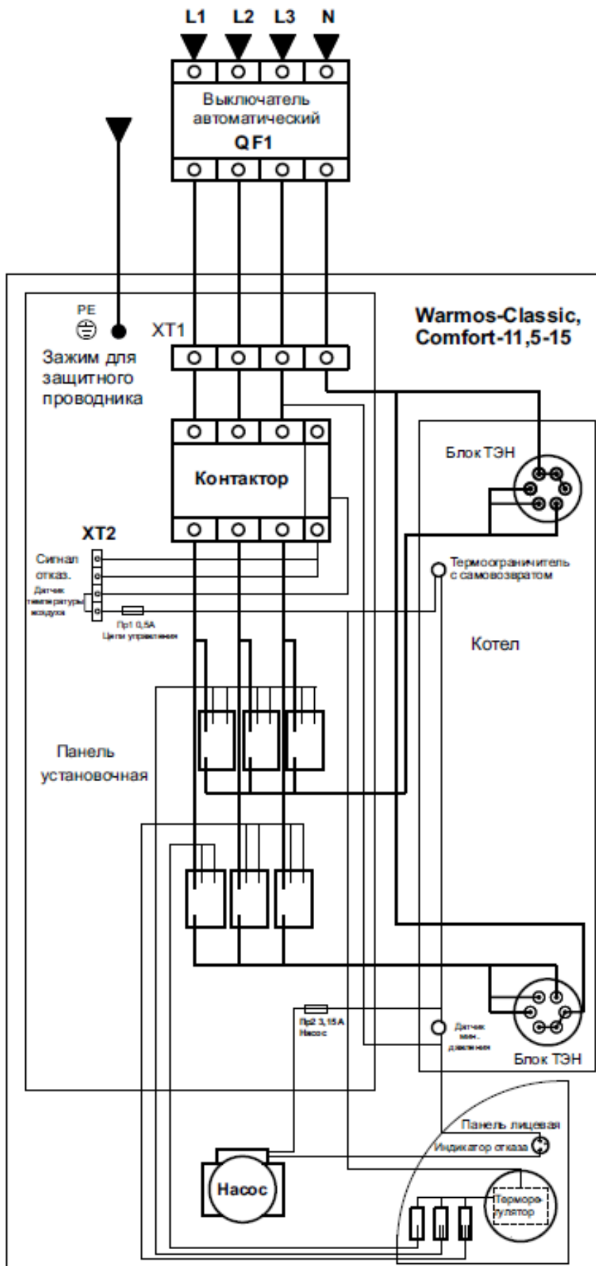
Рисунок 7. Подключение приборов Warmos CLASSIC, Warmos COMFORT – 11,5-15 кВт
