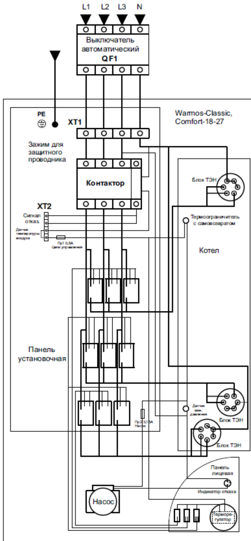
Рисунок 8. Подключение приборов Wamos CLASSIC, Wamos COMFORT – 18-27 кВт
