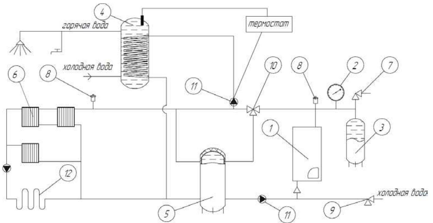
Рисунок 4. Возможная схема системы отопления и ГВС
