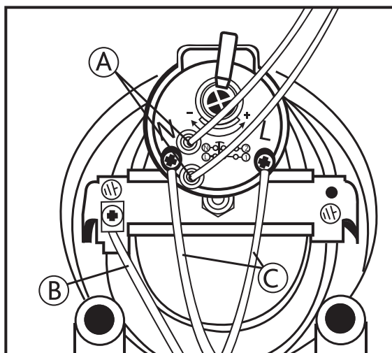
Автоклавний фланець
